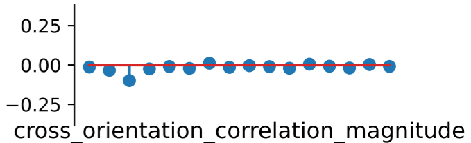
magnitude_std
